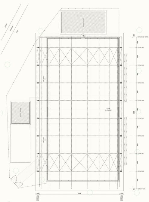
Pianta progetto esecutivo
