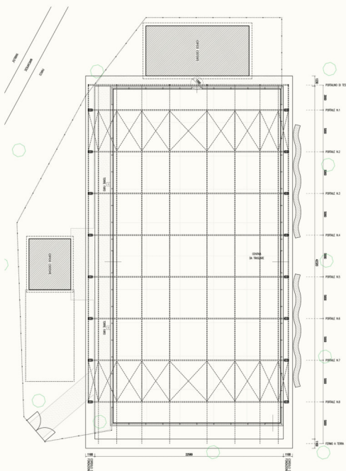
Pianta progetto esecutivo
